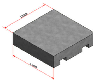
SKR-015-2,5B Bloque de hormigón 1000Kg
