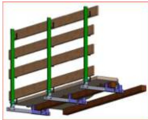
Fijación lateral a vigas de madera
