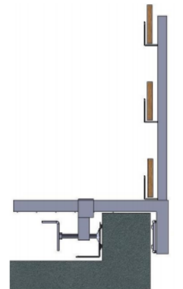
FIJACIÓN A MURETE
