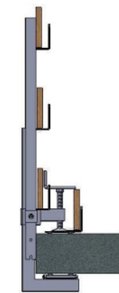
FIJACIÓN A LOSA
